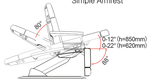
Simple Armrest
